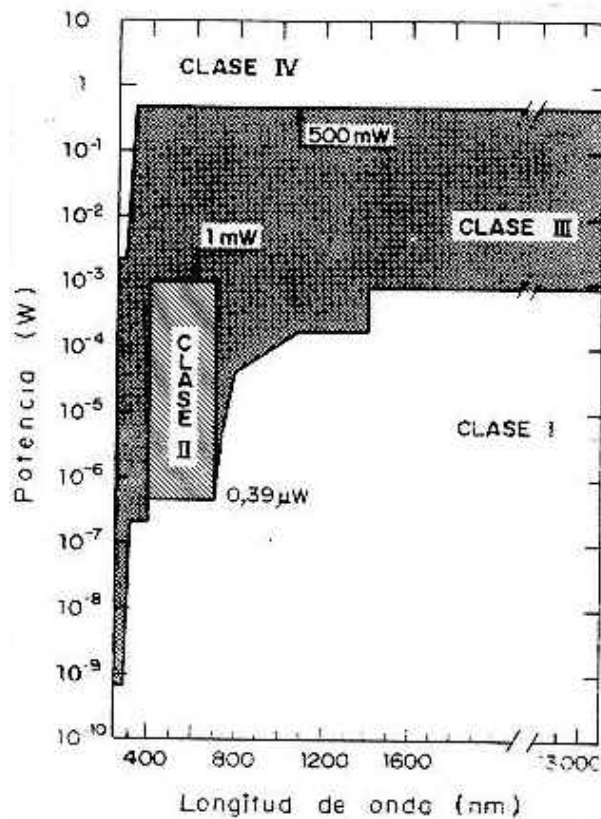
Fig. 4: Clasificación de láseres de emisión continua del BRH en 1978
