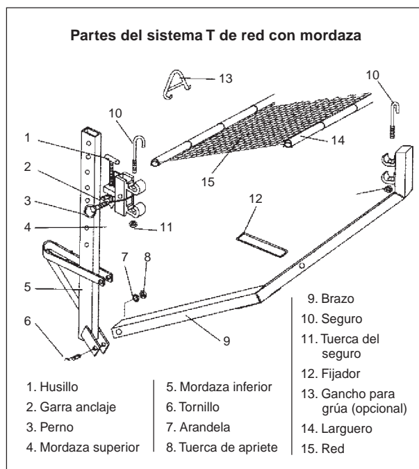
Figura 5. Red de seguridad. Componentes del sistema T
